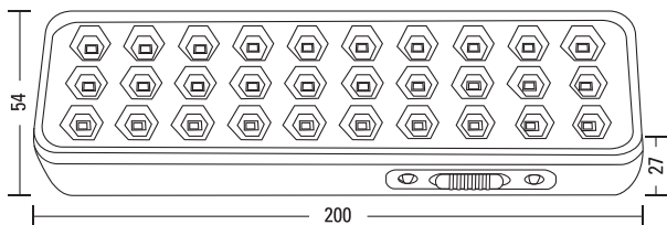
Рис. 1. Габаритные и установочные размеры BACKUP-150
