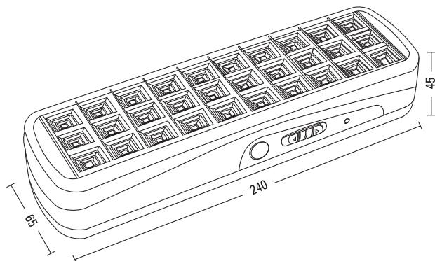
Рис. 2. Габаритные и установочные размеры BACKUP-250 / 250P
