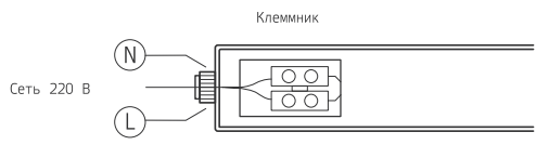
Рис. 2. Схема подключения светодиодного светильника Universal к сети 220 В
