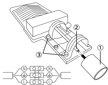
Рис. 1. Монтаж светильника
