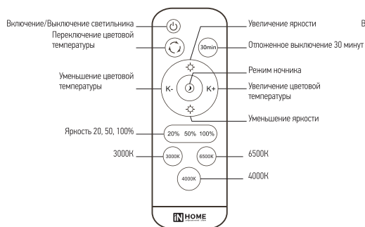
Рис. 1 Управление светильником
